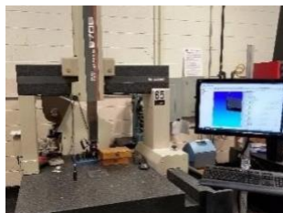
MITUTOYO B706
